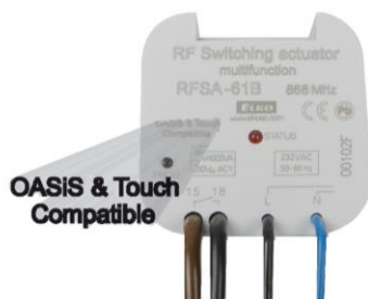
Obr. 10: Označení RF prvků nápisem "OASIS & Touch Compatible".
