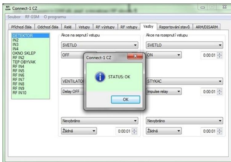
Obr. 48: Položka "Diagnostika" – stav jednotky RFGSM-220M.
