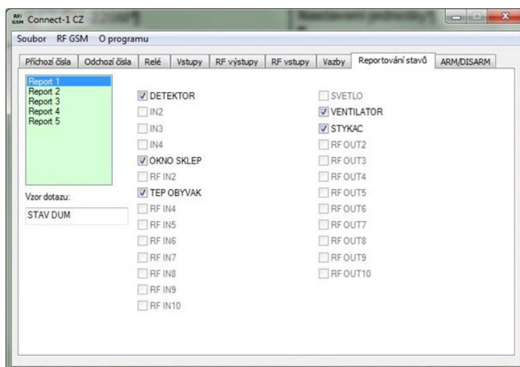
Obr. 21: Záložka "Reportování stavu" – zadání vzoru dotazu a výběr vstupů a výstupů pro reportování stavu.
