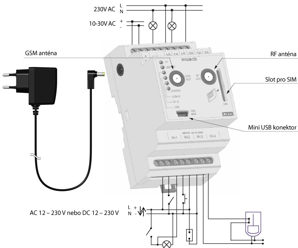
Obr.2 Zapojení vstupů a výstupů RFGSM-220M.
