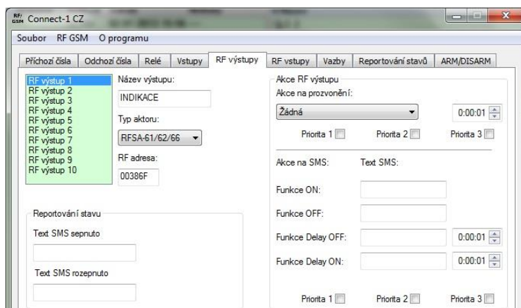
Obr. 35: Záložka "RF výstupy" – zadání RF prvků, které budou použity pro indikaci zapnutí / vypnutí střežení zóny a pro signalizaci poplachu.
