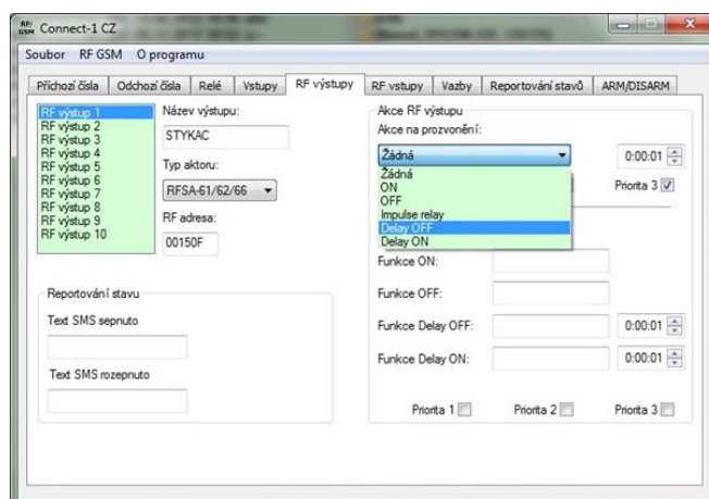
Obr. 12: Záložka "RF výstupy" – výběr akce na prozvánění jednotky RFGSM-220M.
