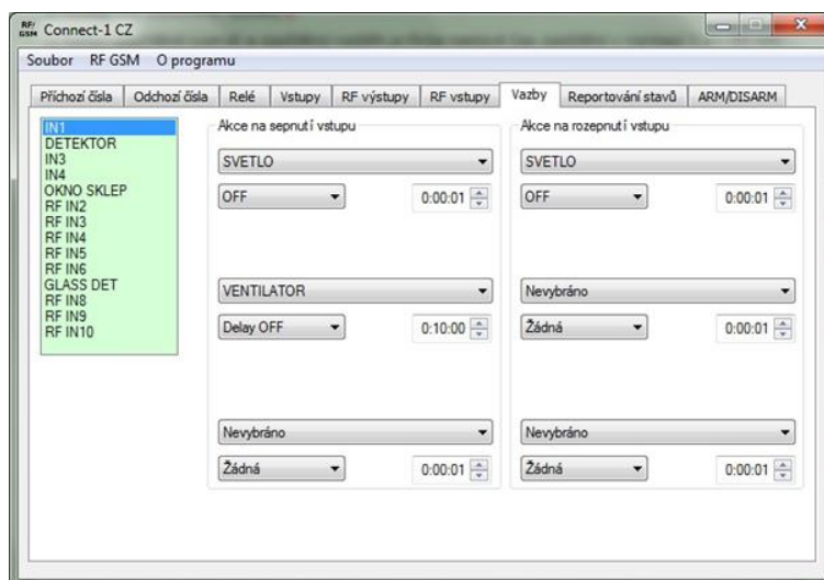
Obr. 20: Záložka "Vazby" – výběr akcí na lokálních / RF výstupech.
