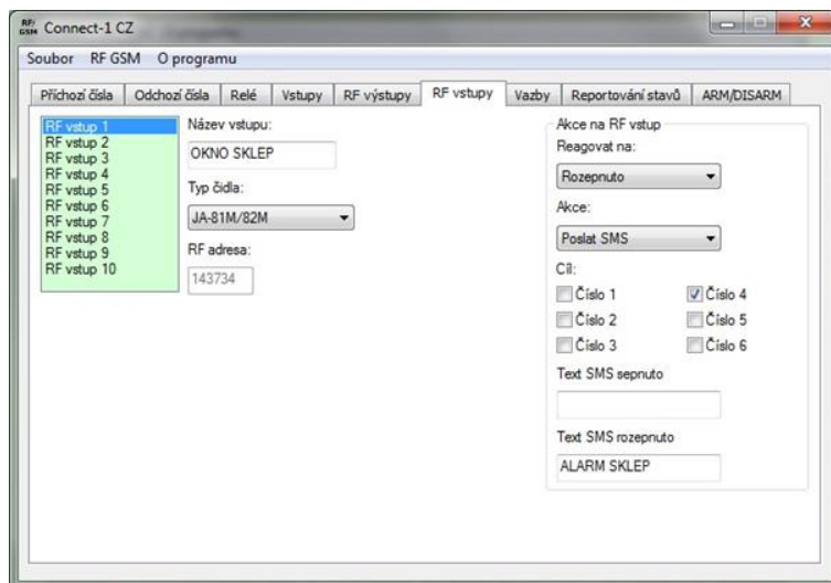
Obr. 19: Záložka "RF vstupy" – výběr změny na vstupu, na jejímž základě budou vysílány SMS.
