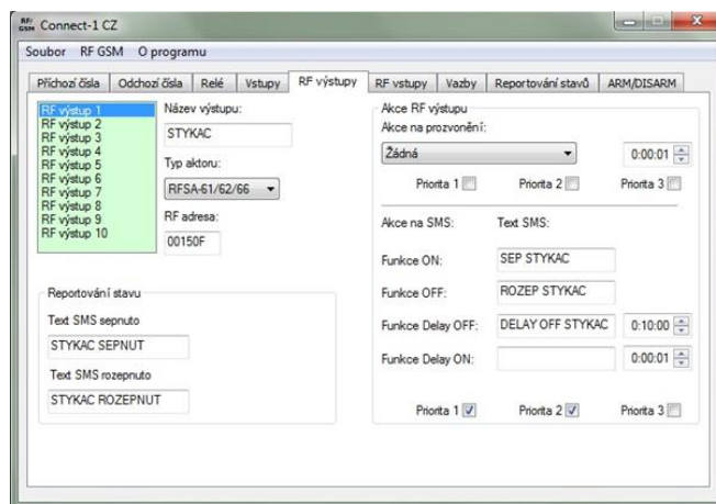
Obr. 13: Záložka "RF výstupy" – výběr akce na přijatou SMS a volba textu pro reportování stavu RF výstupů.
